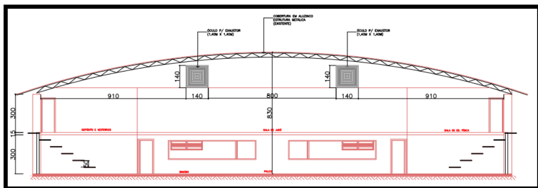
Desenho 01: Abertura de 2 (dois) Óculo para Exaustores
