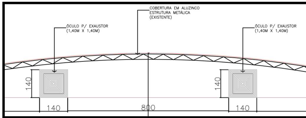
Desenho 02: Abertura Óculo para Exaustores
