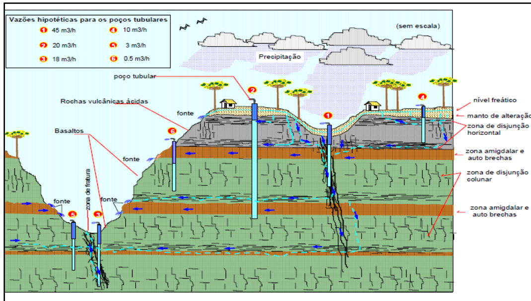
Fig. 3— Modelos de perfis encontrados na região de abrangência do Aquífero Serra Geral. Importância do reconhecimento das fraturas na superfície. Existem duas possibilidades de fluxo d'água no poço que são as fraturas e os contatos de derrames. Assim poços perfurados fora dos sistemas de fraturas podem apresentar vazões quando interceptam a zona vesicular no contato de derrames vulcânicos.
