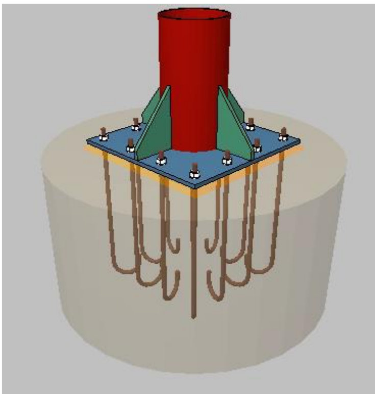
Figura 05 – Chumbadores, enrijecedores e placa base
