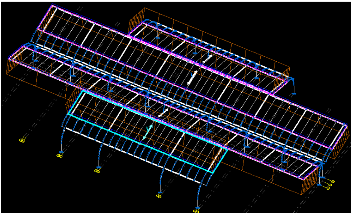
Figura 03 – Cargas aplicadas na estrutura metálica
